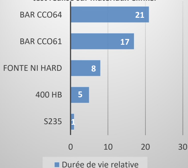
Comparatif théorique de performances test réalisé sur matériaux Clinker
