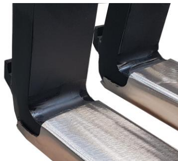
Détail du talon de fourche selon norme NF EN 1755 (ATEX)
