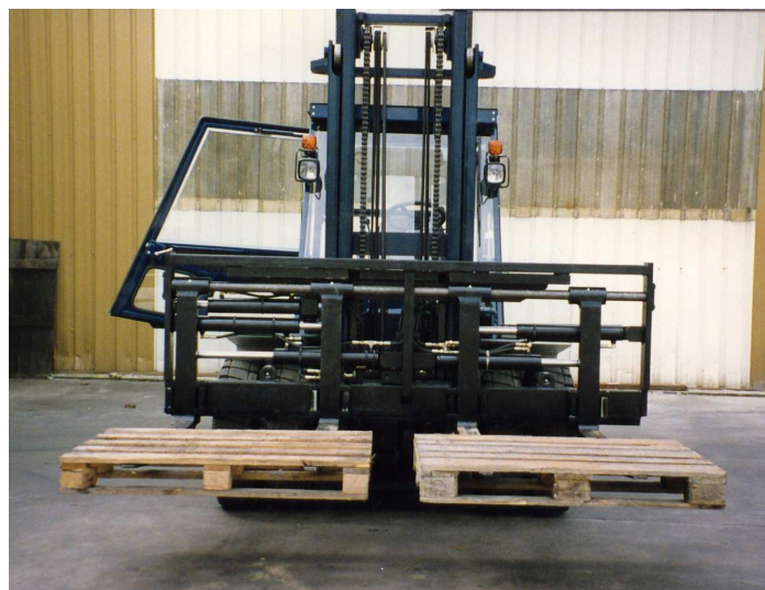
Triple TDL intégré avec positionneur de fourches Grande visibilité
