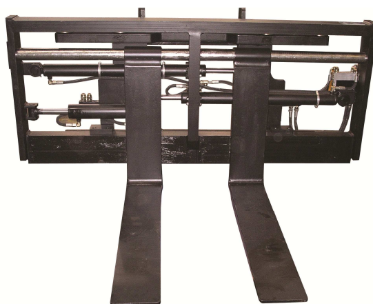
TDL constant avec positionneur de fourches (3 vérins)
