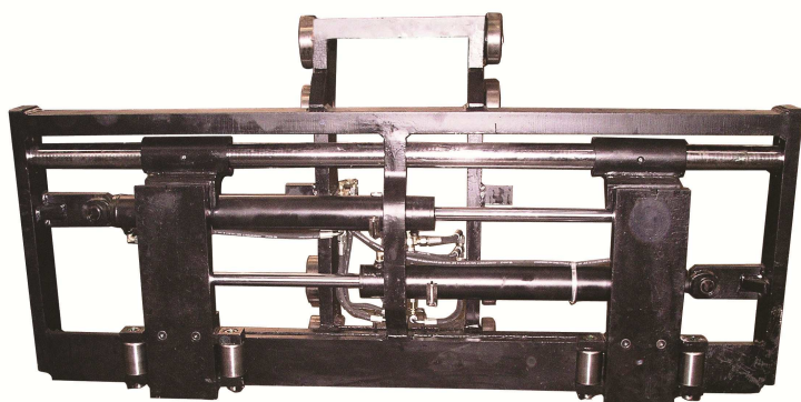
TDL progressif avec platine à dépose rapide (2 vérins)
